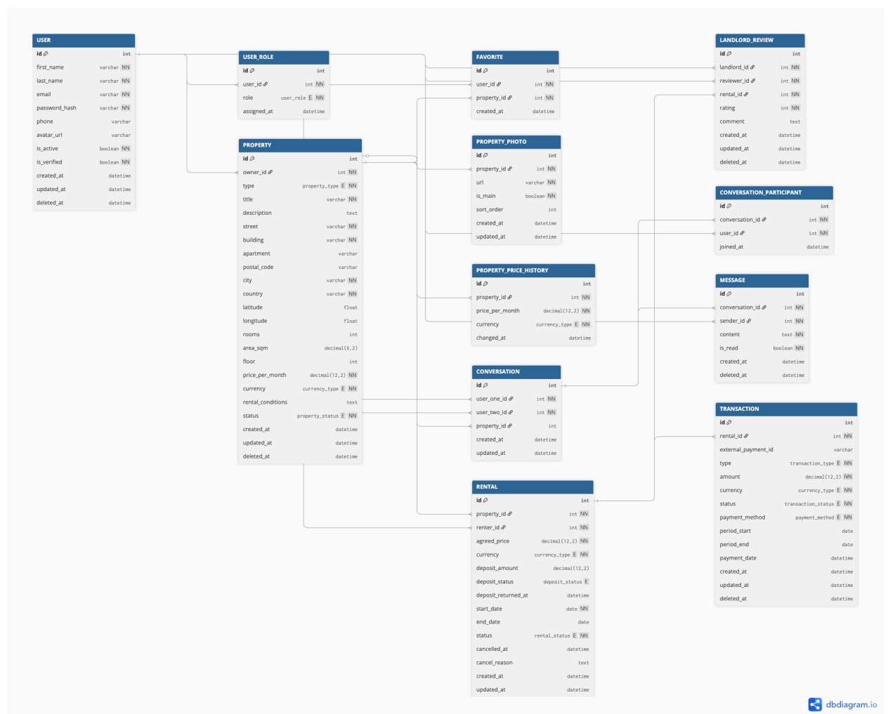
Рис. 1. ER-диаграмма сервиса для аренды недвижимости
